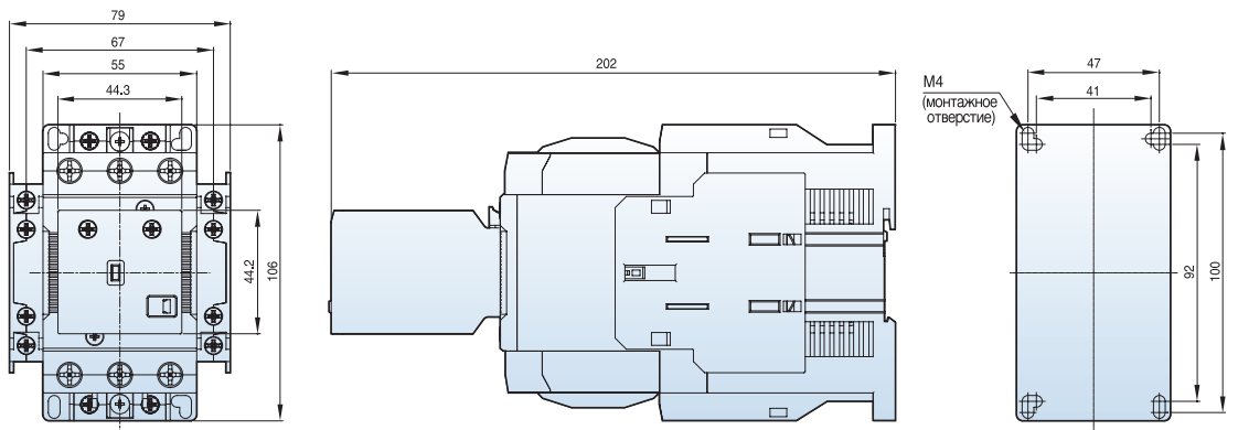
MC-50a~65a DC
