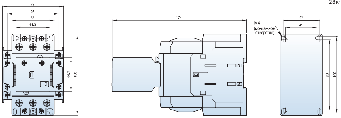
MC-50a~65a AC
